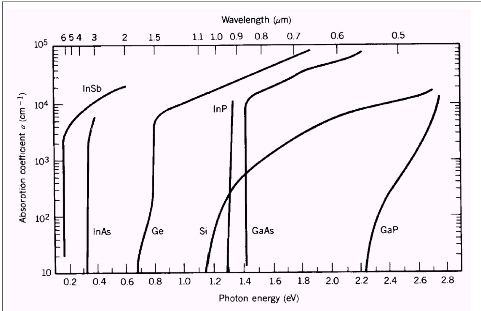
Abbild 1: \alpha - Materialwerte verschiedener Halbleitermaterialien zum Einsatz in Fotodetektoren
